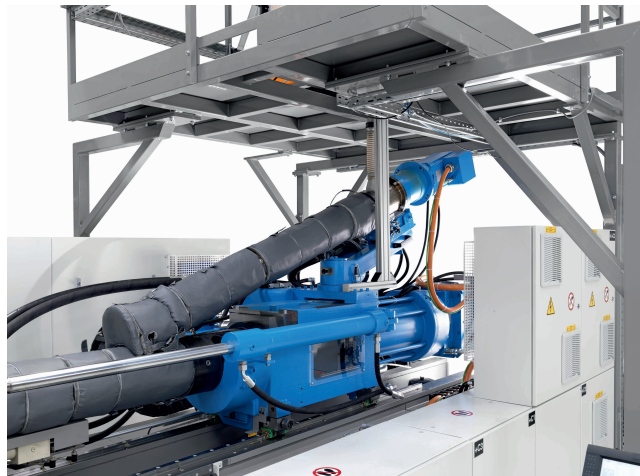
Bild 1. Beim DCIM-Verfahren compounding ein Einschneckenextruder mit direkter Verbindung zur Plastifiziereinheit. © KraussMaffei
