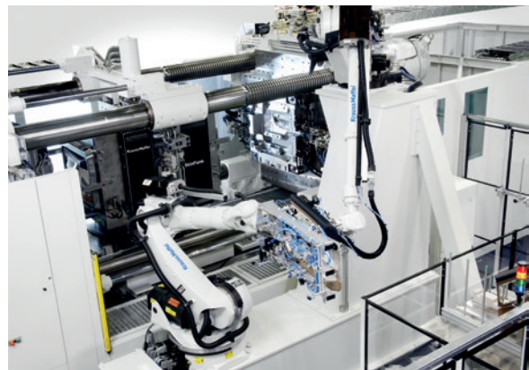
MX-Baureihe als Dreikomponenten-SpinForm-Technologie (Wendeplatte) ausgeführt.
